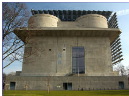
BHKW-Kompaktmodul GG 530 BHKW-Kompaktmodul GG 237 Energiebunker Hamburg-Wilhelmsburg
