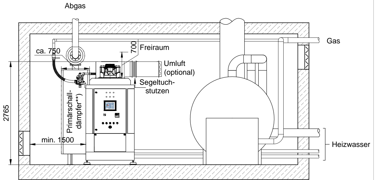
Ansicht BHKW Abluft
