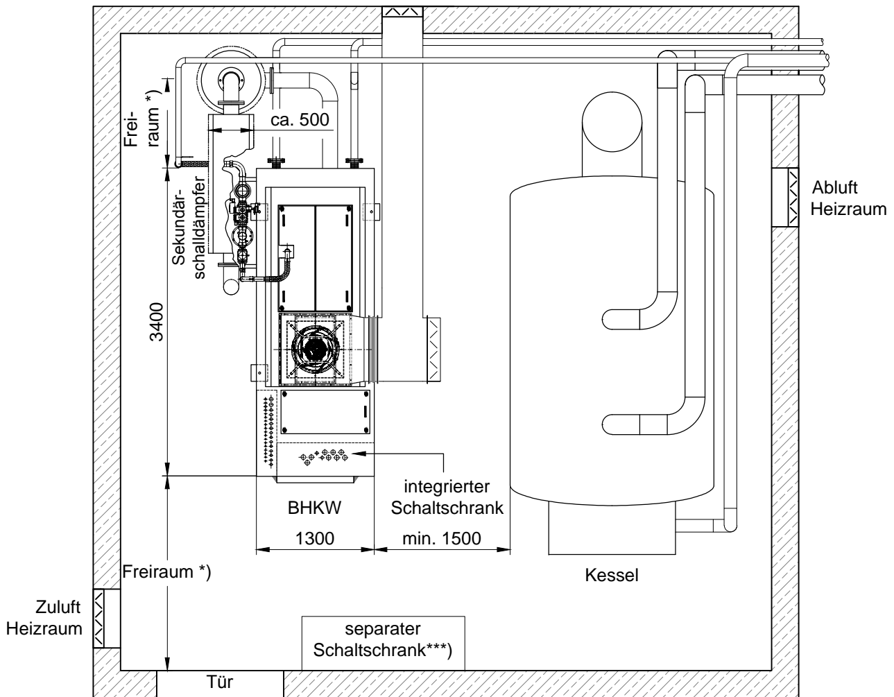
Türbreite min. 1400 mm Türhöhe min. 2350 mm Draufsicht
